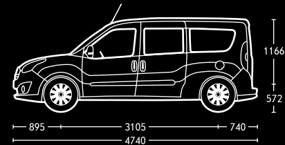
Combi (N1) cu geam cu ampatament lung și plafon standard.
