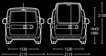
Tour și Cargo cu plafon standard sau înălțat.
