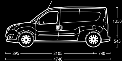
Cargo cu ampatament lung și plafon standard.
