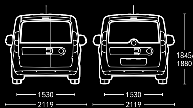
Tour și Cargo cu uși spate asimetrice sau hayon.
