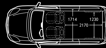
Cargo cu ampatament lung și plafon standard.
