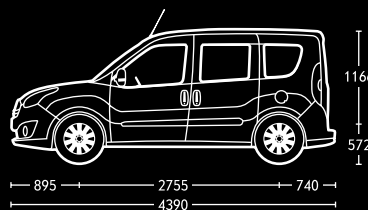
Tour și Cargo cu geam cu ampatament și plafon standard.
