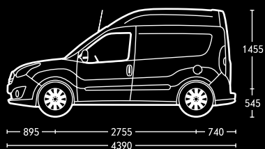
Cargo cu ampatament standard și plafon înălțat.
