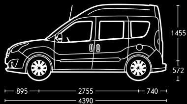
Tour și Cargo cu geam, cu ampatament standard și plafon înălțat.
