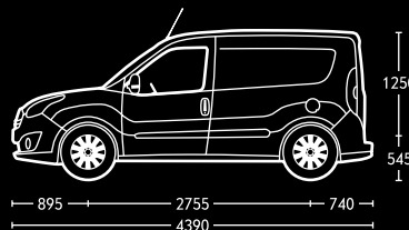
Cargo cu ampatament și plafon standard.
